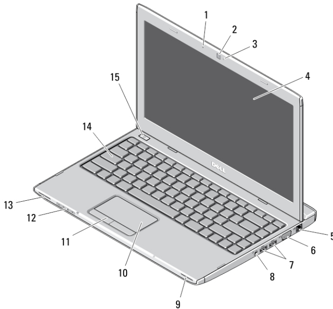
圖 1. 前視圖
